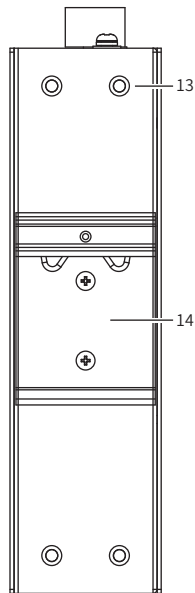
TL-SG2005工业级 后面板示意图
