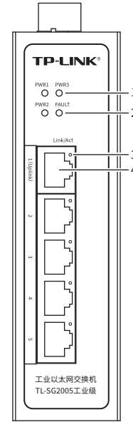
TL-SG2005工业级 前面板示意图
