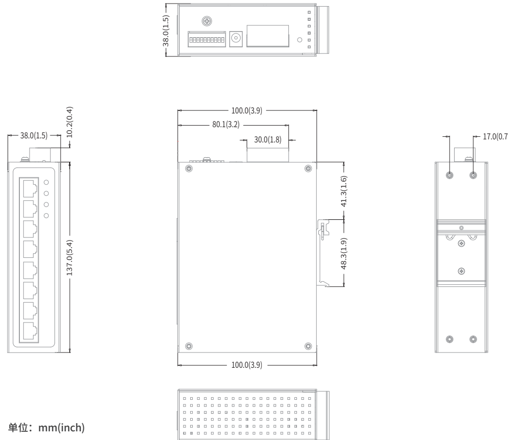
TL-SG2005工业级
