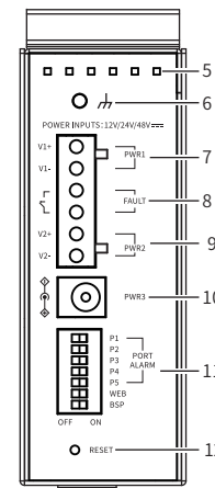
TL-SG2005工业级 上面板示意图
